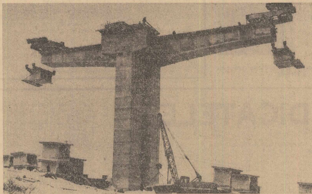
O imagine de la lucrările de montaj a elementelor prefabricate ce vor forma suprastructura marelui viaduct gălățean, prin intermediul cărui drumul de acces între oraș și combinat va fi scurtat cu circa 12 kilometri. Foto: FLORIN ȘTEFĂNESCU
