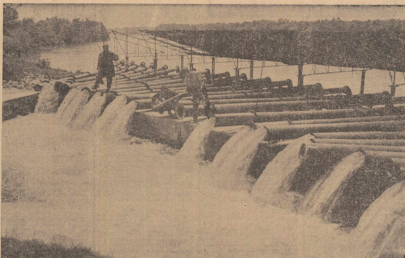
Stația de pompare a sistemului de hidroameliorații Drăgănești-Ort
