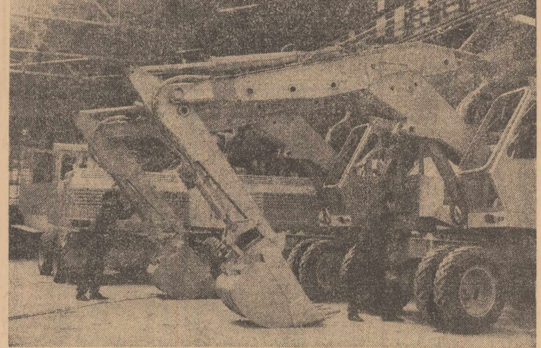
Producția uzinei de utilaj greu „Progresul” din Braila cuprinde o gamă variată de tipuri de excavatoare. Unul dintre acestea: Excavatorul P-601, pe care-l vedeți în fotografia noastră. Dotat cu un echipament care permite utilizarea sa la o multitudine de lucrări pentru construcții, acest vâslor al uzinei brailene se numără printre exponatele reprezentative ale țării noastre la expozițiile și târgurile internaționale.
