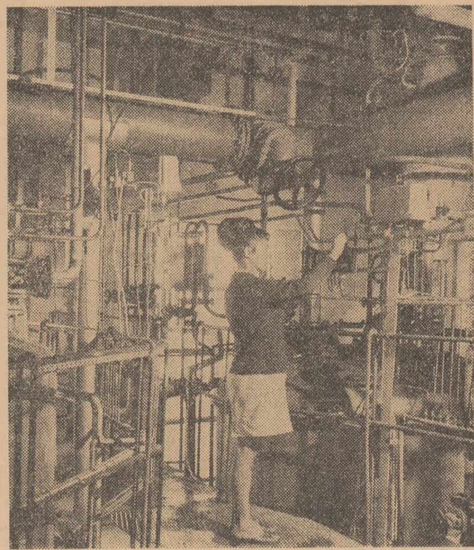
În cadrul Combinatului alimentară „7 Noiembrie” din Arad a intrat în producție noua fabrică de drojdie furajeră cu o capacitate de 1920 de tone pe an. Beneficiind de un înalt grad de automatizare, cu un indice de utilizare a spațiului foarte ridicat, fabrica de drojdie furajeră produce în momentul de față 6 tone pe zi. În clădirea instalată de fermentare a fabricii de drojdie furajeră.
