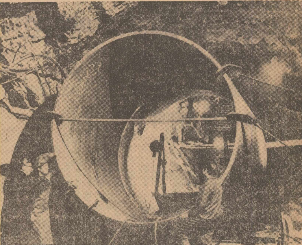
Lucrări de montaj la virolele conductei din galleria forțată a centralei hidroelectrice subterane de la Ciungnet.
