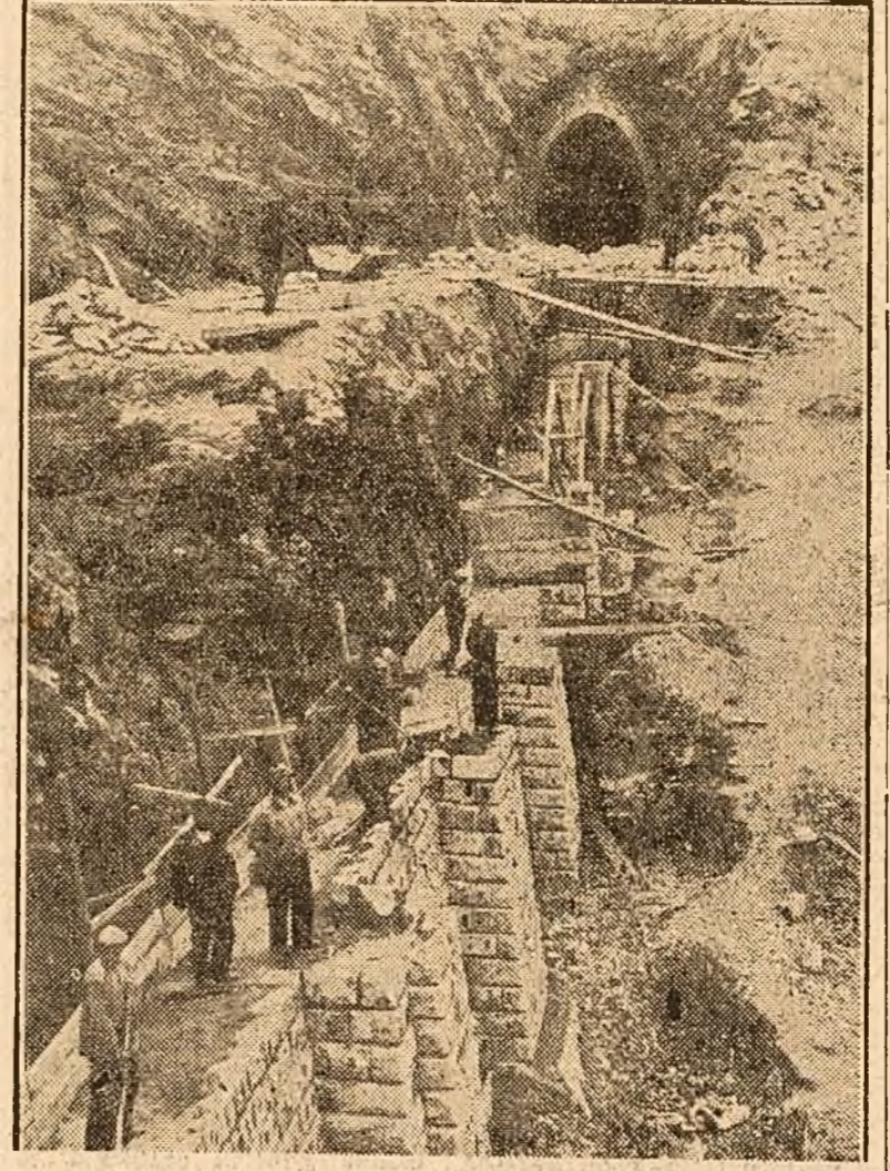
Postamentul unui viaduct în prima fază de lucru pe linia Bumbesti-Livezeni
