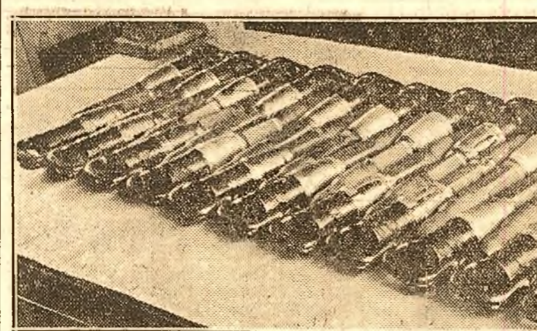
O serie de ciocane de abataj, fa bricate de secția „Sculărie” a uzinelor Reșița.
