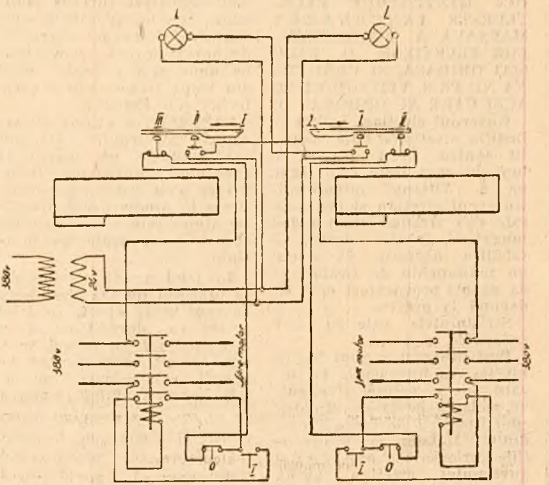
Pentru ca să asigure buna funcționare a celor două strunguri la care lucrează, tov. Șerbănescu N. a instalat un dispozitiv electric de semnalizare și oprire.
