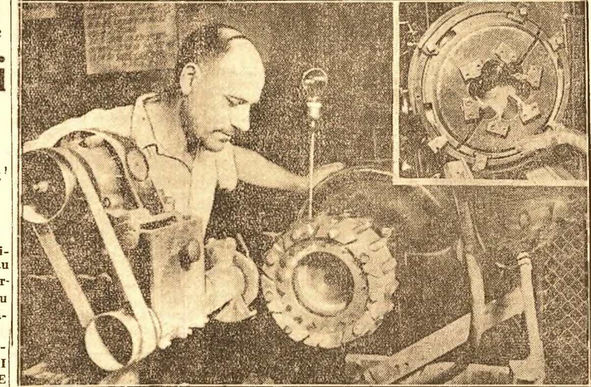
Tov. N. Șerbănescu, lucrând la unul din cele două strunguri la care a aplicat noul dispozitiv conceput de el, dispozitiv de care sunt prinse cele 18 bacuri. În medallion: dispozitivul vechi pe care puteau fi fixate — în interior — numai 6 bacuri
