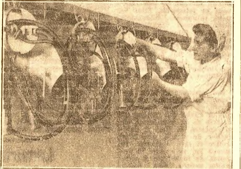
În colhozul „Crasnăi Partizan” vechile sunt mulate cu ajutorul aparatelor electrice. Fiecare mulgătoare are în primire un aparat pe care îl ține în cea mai perfectă stare.
