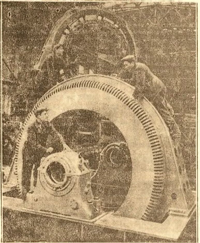
La uzina „Electrosila” din Leningrad, întrecerea în cinstea zilei de 7 Noiembrie este în toi. Urășul generator din ciuj, destinat unei fabrici de cauciuc sintetic, va fi terminat în ajunul sărbătorii.
