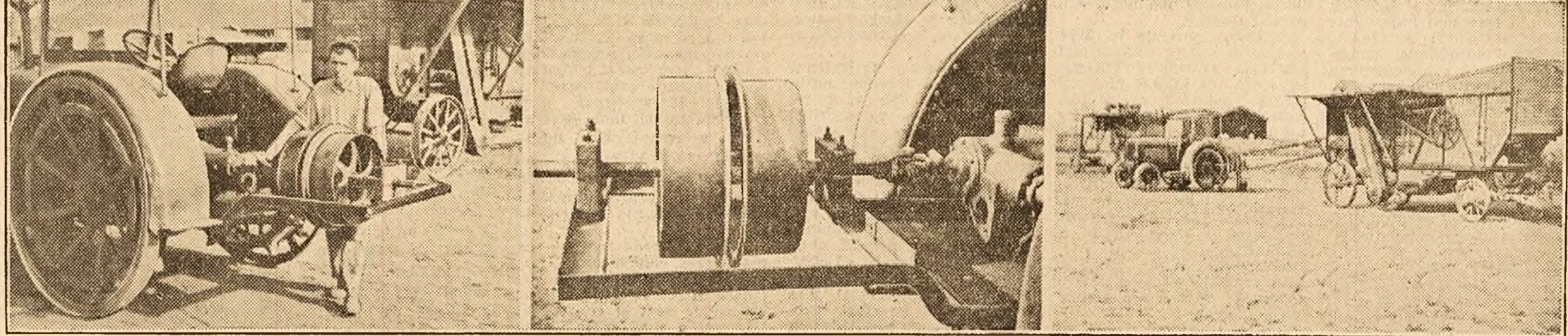
Tovarășii Coconoiu Gheorghe și Saicu Dumitru mecanici dela S.M.T. Băilești-Dolj au construit un dispozitiv cu ajutorul căruia pot fi cuplate două batoze la un singur tractor, inovație care, pusă în practică, poate reduce la jumătate numărul tractoarelor necesare treierii, restul putând fi întrebuințate la desmăturări.
