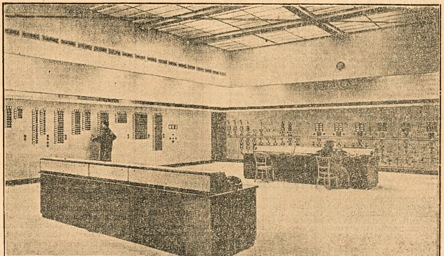
La marea centrală electrică „7 Noiembrie” dela Inota în R. P. Ungară, zeci de agregate și aparate complicate sunt mânuite, după cum se vede mai sus, numai de doi oameni.
