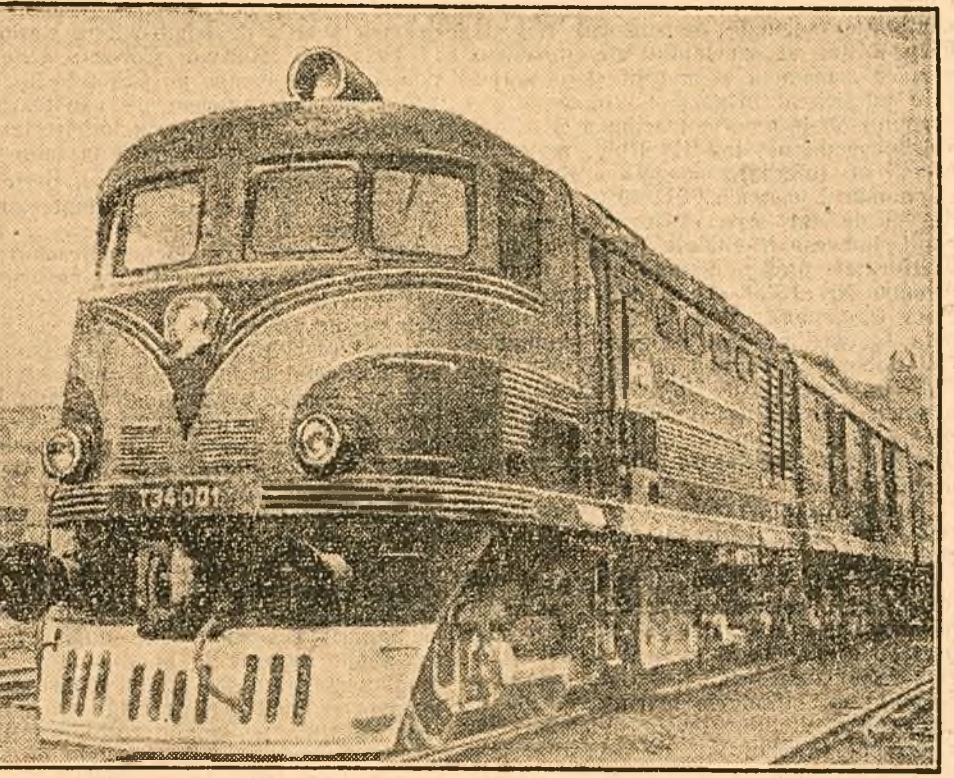
Industria socialistă a Uniunii Sovietice înzestrează transportul pe calea ferată cu mijloace tehnice tot mai desăvârșite: locomotive electrice, locomotive „Diesel“ și locomotive cu generator de gaze. Unul din cele mai perfecționate și puternice tipuri de locomotivă este locomotiva „T.E.-4“, cu o capacitate de 2000 cal putere, care folosește drept carburanți în proporție de 75% gaze produse în corpul locomotivelor prin arderea antracitului, precum și 25% carburanți lichizi. „T.E.-4“ folosește de trei ori mai puțin cărbune decât o locomotivă obișnuită. În clișeu: noua locomotivă „T.E.-4“.
