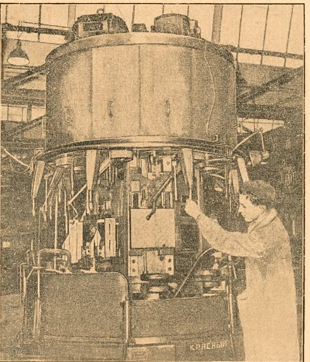
Uzina de tractoare din Orașul Stalin a fost înzestrată în ultimii ani cu noi mașini și utilaje de înaltă tehnicitate sosită din Uniunea Sovietică. În clăuse: strungarul frunțas în producție Hans Zoor lucrând la mașina semiautomată „Crasnăi Proletarii“. La această mașină, deservită de un singur muncitor, se strunjește deodată, la ambii butuci, 6 corpuri de role pentru șenilele de tractoare.
