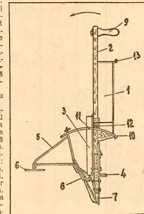
Semănătoarea manuală S.M.-1
