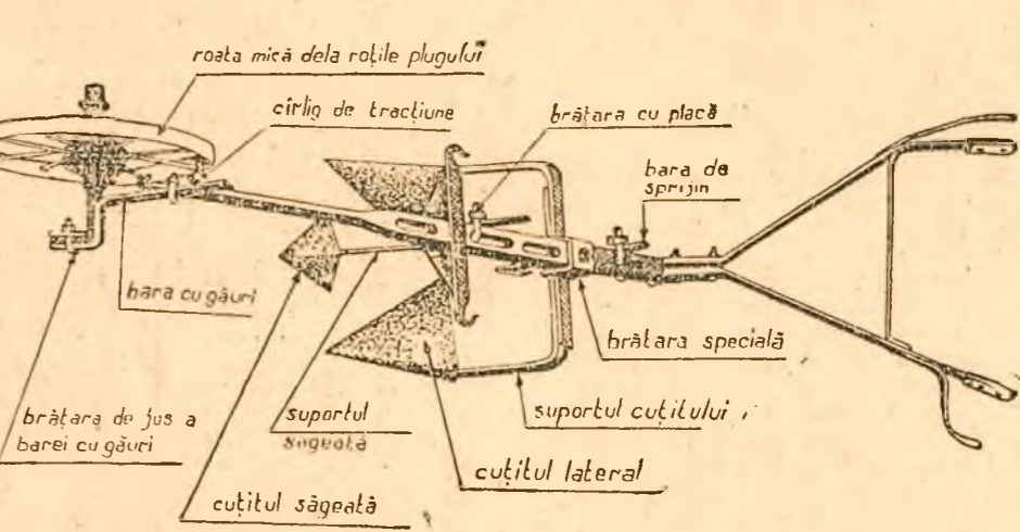
În clipșu: un model de prășitoare făcută prin transformarea unui plug de tracțiune animală.
