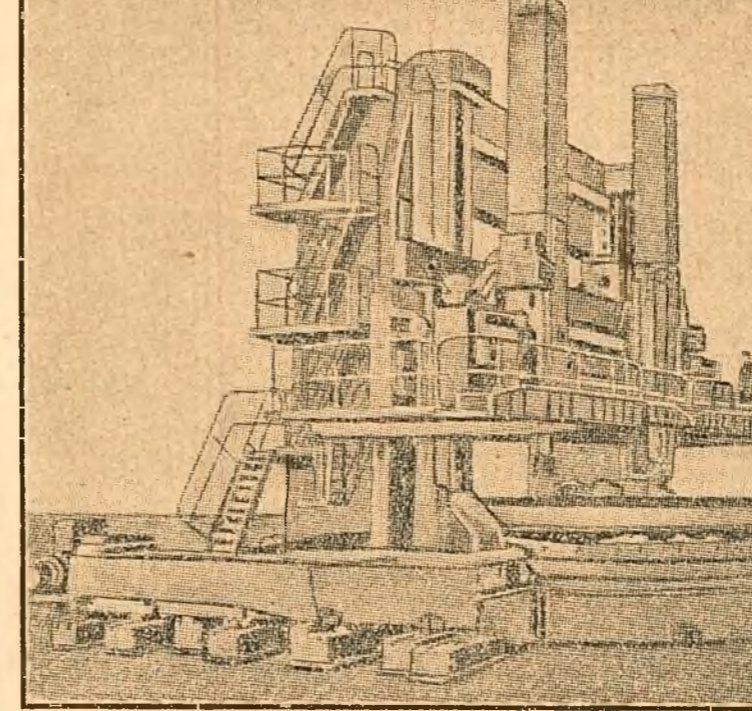
Sub conducerea constructorului-șef I. V. Hromov, colectivul Biroului de construcții al Ministerului Construcțiilor de Mașini al U.R.S.S. a construit strungul MK-159, al cărui platou are un diametru de 8750 mm. Strungul prelucrează piese cu diametrul de 9200 mm și cu o greutate care ajunge pînă la 170 tone. În clișeu: Strungul universal carusel MK-159.
