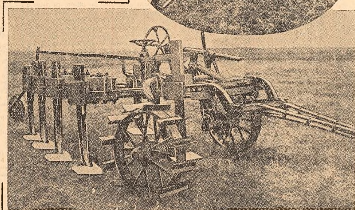
În clișeu: plugul P-5-35 adaptat pentru executarea arăturii în cadrul experimentării sistemului agrotehnic T. S. Malțev. În medalion: Tractoristul Ștefan Todici executînd arătura la adîncime de 40-50 cm. cu ajutorul puternicului tractor sovietic „Stalin” și al plugului P-5-35 adaptat acestui lucrări.
