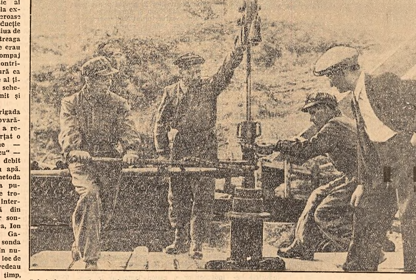
Sub îndrumarea inginerului tehnolog Ion Istrate, o echipă de sonderi din brigada de intervenție condusă de tov. Petre Moise pune în pompaj forțat sonda nr. 2.
