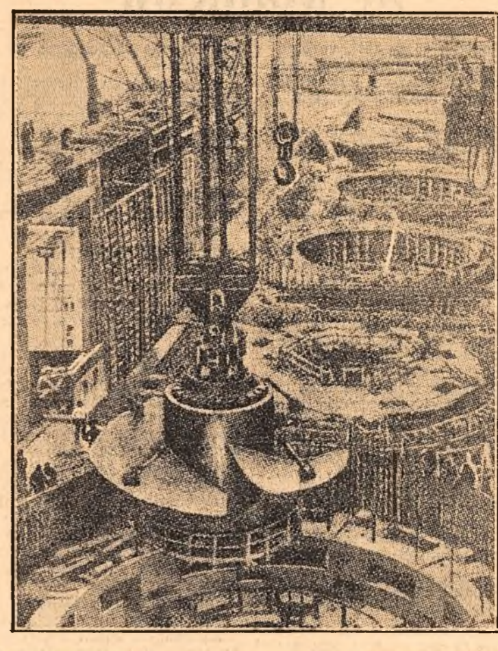
După aproape 2 ani de lucrări pregătitoare, constructorii nodului hidroenergetic de la Kahovka au reușit într-un timp record — în numai 2 zile, față de 12 zile cît prevedea planul — să închidă complet abia Niprului și să îndrepte apele fluviului pe o nouă abie, spre barajul devorator de beton armat. Pentru nevoile navigației au fost puse în funcțiune ecluzele. La începutul lui iulie 1955, între malurile Niprului mai rămăsese o trecere lungă de 230 metri și la sfîrșitul lui mai rămăsese o trecere lungă de 17 metri. Pe podul de porțonare, construit peste această trecere, au circulat fără intreruperi, zi și noapte, siruri și siruri de camioane basculante, aruncînd în fluviu balturi mari și blocuri de beton. Toată, drage refulante puternice împingeau fără încetare, prin 4 conducte cu debit mare, cantități uriașe de pulpă — pămînt amestecat cu apă — sedimentîndu-le printre blocurile și bolovanii ce urmasă să bazeze calea apelor Niprului. Alături de ele, la deplasarea marilor cantități de pămînt, au acționat și 4 hidro-monitoare puternice. Rîmul lucrărilor de sedimentare a atins 100.000 m 3 de pămînt deplasat în 24 ore.
