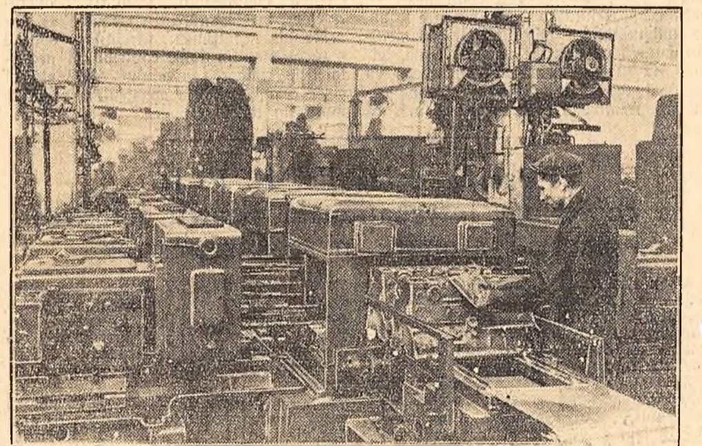
La uzina de automobile „Molotov” din orașul Gorki se instalează noi linii de mașini automate. În clăuse: Liniă automată pentru prelucrarea părții frontale a blocului de motor, în prima fază a operației.
