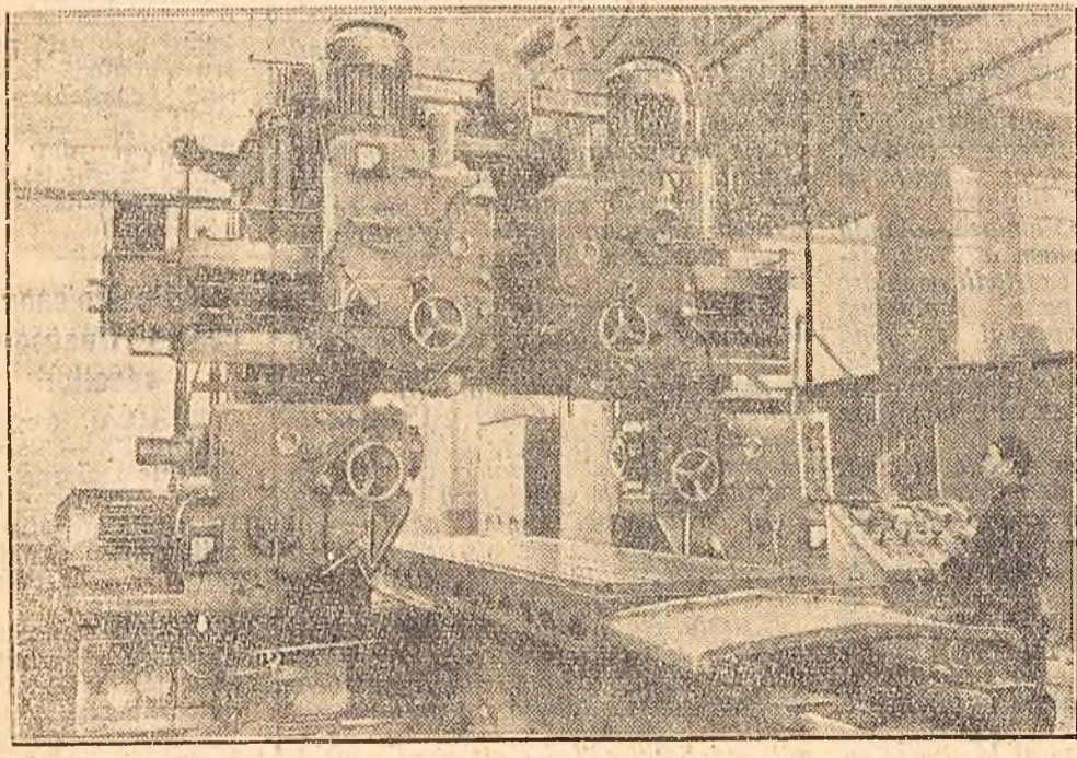
Uzina „Lenin-Kolli” din Leningrad produce puternice mașini de frezat. De cîrînd ea a livrat o nouă mașină de frezat longitudinală cu patru axe. Greutatea mașinii se ridică la 64 tone, iar lungimea ei este de 11 metri. În clăuse: N. Lobanov, șeful brigăzii de montaj, face rodajul noii mașini.
