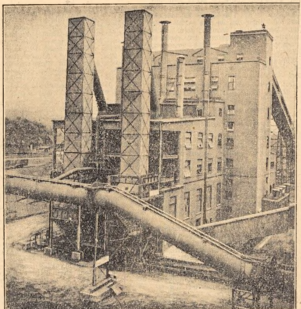
Fabrica de aglomerare de la combinatul siderurgic „Gh. Gheorghiu-1” din Humedora — una din marile construcții ale cincinalului, realizată cu itorul Uniunii Sovietice — are o deosebită însemnătate pentru dezvoltarea industriei terestre din țara noastră. La ridicarea acestei fabrici s-au turnat 60.000 metri cubeton armat, s-au zidit peste 7.000 metri cubi cărămidă, s-au executat săpături carechivă-lază cu săpăturile unui tunel de 4 km. etc. Întregul proces tehnologic este manizat. Transportul prafului de minereu de fier și de coacs se face pe benzii transportoare
