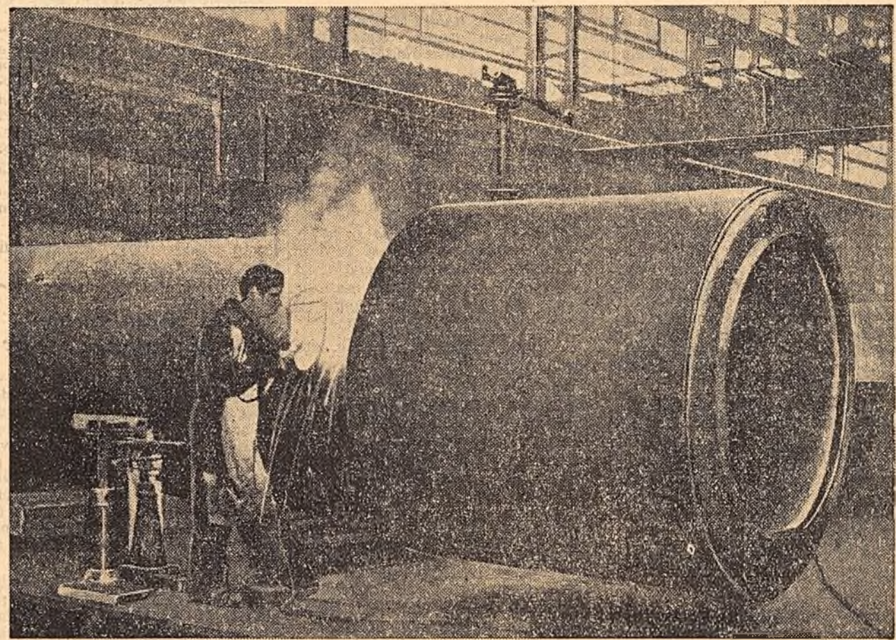
La Complexul C.F.R. „Grișuța Roșie” din Capitală a început de curînd construirea cazanelor de locomotive asamblate prin sudură electrică, în loc de nițuire. Acest procedeu a fost studiat și introdus de tov. Dumitru Croicu, șeful secției a III-a cazanerie, care s-a specializat în Uniunea Sovietică.
