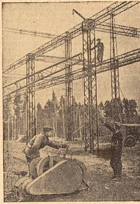
Un aspect al instalării linilor de transport de energie electrică Irkutsk-Bratsk.
