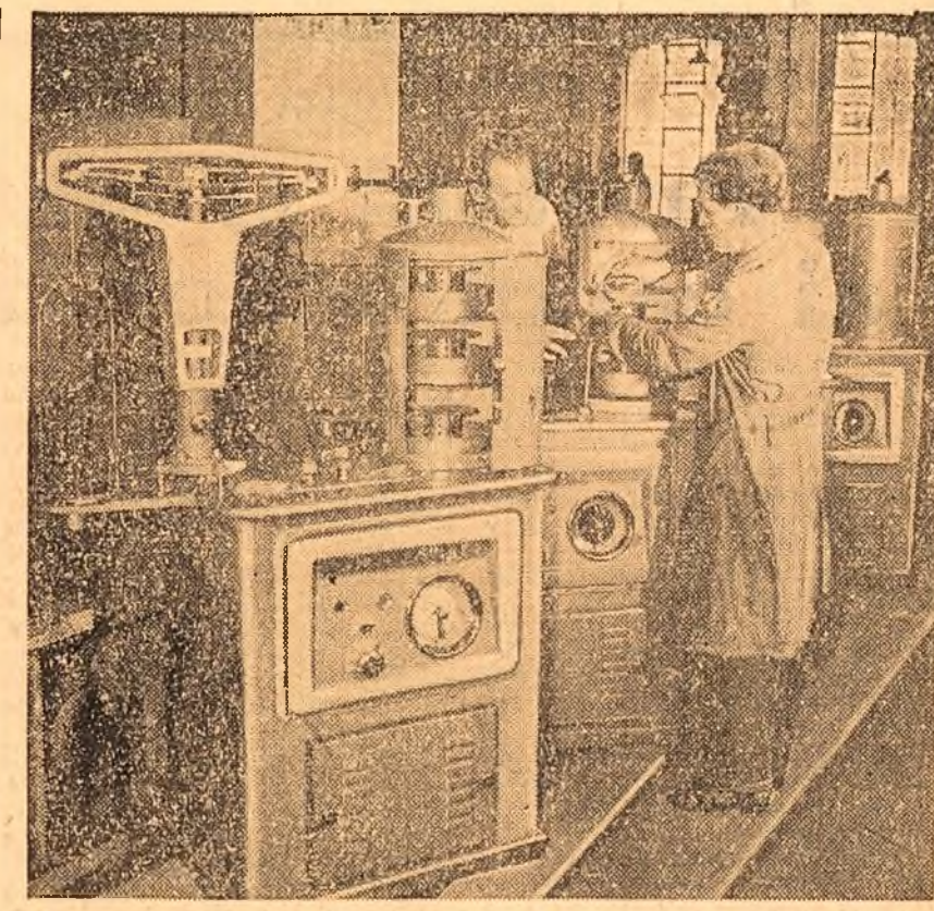
Un nou aparat de măsură și control a fost înscris nu de mult în catalogul produselor fabricate în țara noastră. Cu ajutorul acestui aparat — care se fabrică în prezent la unitatea de aparate pentru laborator și prototipuri a întreprinderii „Tehnometal” din Capitală — se determină ușor gradul de umiditate a materialelor textile. În clișeu: Aspect din timpul montării unui nou aparat.
