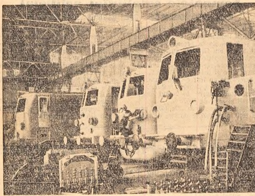
Uzina „L.E.W.” din Hennigsdorf a început producția de locomotive electrice rapide în 1955. Astăzi, ele se exportă în multe țări ale lumii, unde sint bine apreciate. În clipă: Un aspect din hala de montare a locomotivelor electrice.
