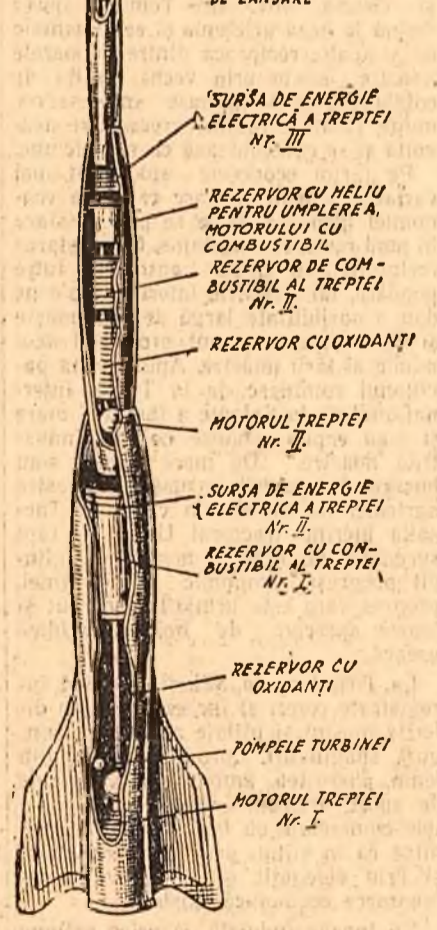
Schema unei rachete în trei trepte pentru lansarea unui satelit artificial
