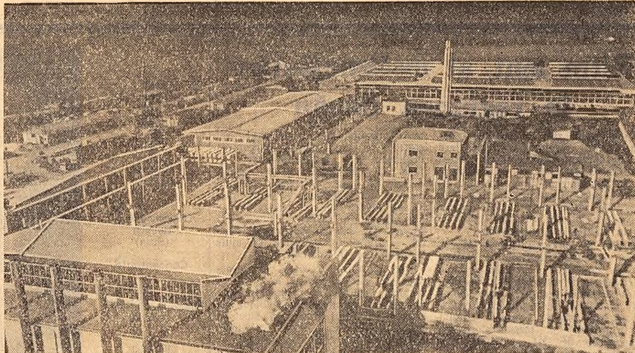
Uzinele „Industria Sirmei” din Cimpia Turzii își schimbă înfățișarea. Pentru lărgirea producției aici a început să se execute noi lucrări. Hale noi de producție, înzestrate cu utilaj modern, se vor adăuga în curând celor existente. În clișeu: un aspect al noilor hale în construcție.
