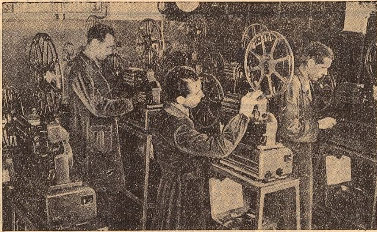
Întreprinderea „Tehnocin” din Capitală a livrat circa 100 aparate de proiecție T-16 pentru înzestrarea unui număr de cluburi și cîmine culturale. Cu ajutorul acestor aparate se pot proiecta filme pe bandă îngustă. În clisur: Înainte de a fi livrate, în întreprindere se face o ultimă probă a aparatelor de proiecție.
