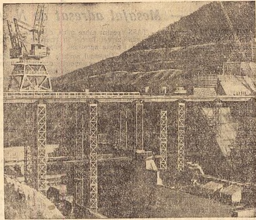
Pe șantierul hidrocentralei „Enver Hodja” s-a terminat construirea celui de-al treilea — ultimul — baraj. Apele rezezi ale râului Mati, care în trecut, în perioadele de revărsare, pricinuiau pagube însemnate unor regiuni întinse, au început să se strîngă într-un lac de acumulare cu un volum de 240 milioane m.c.
