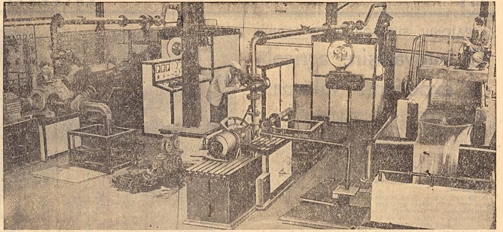
La uzinele „Vasile Roașă” din Capitală a intrat în funcțiune o instalație la care se examinează și probează pompele centrifugale și axiale produse de acest colectiv. Utilajele, ca și proiectul de execuție, s-au realizat în întregime în uzină. În clădire: Noua instalație de probare a pompei. (Foto: GH. VINȚILA)
