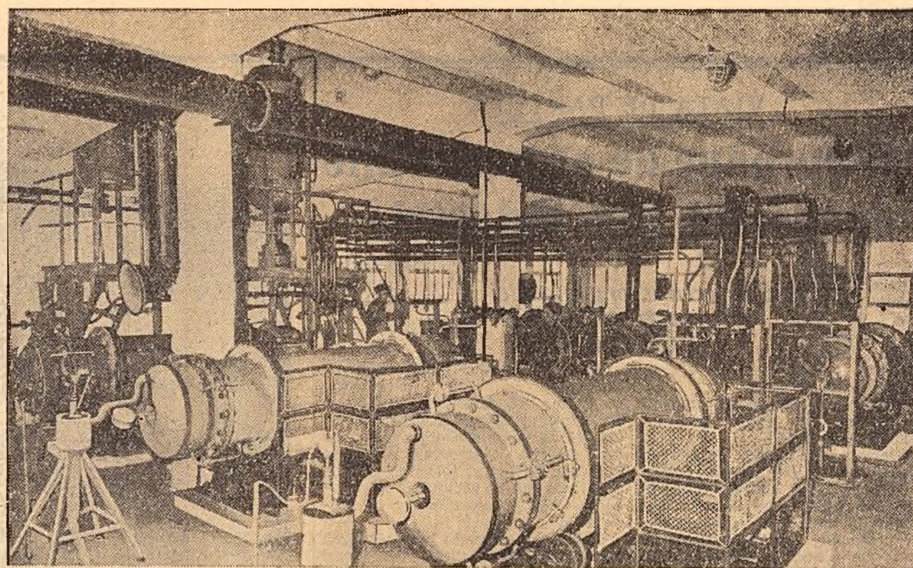
La Combinatul chimic nr. 2 Tirnăveni a intrat în funcțiune anul acesta noua fabrică de polimerizare de vinil, înzestrată cu utilaj fabricat în țară. În clișeu: Aspect din secția de polimerizare. (Foto: GH. VINȚILA)
