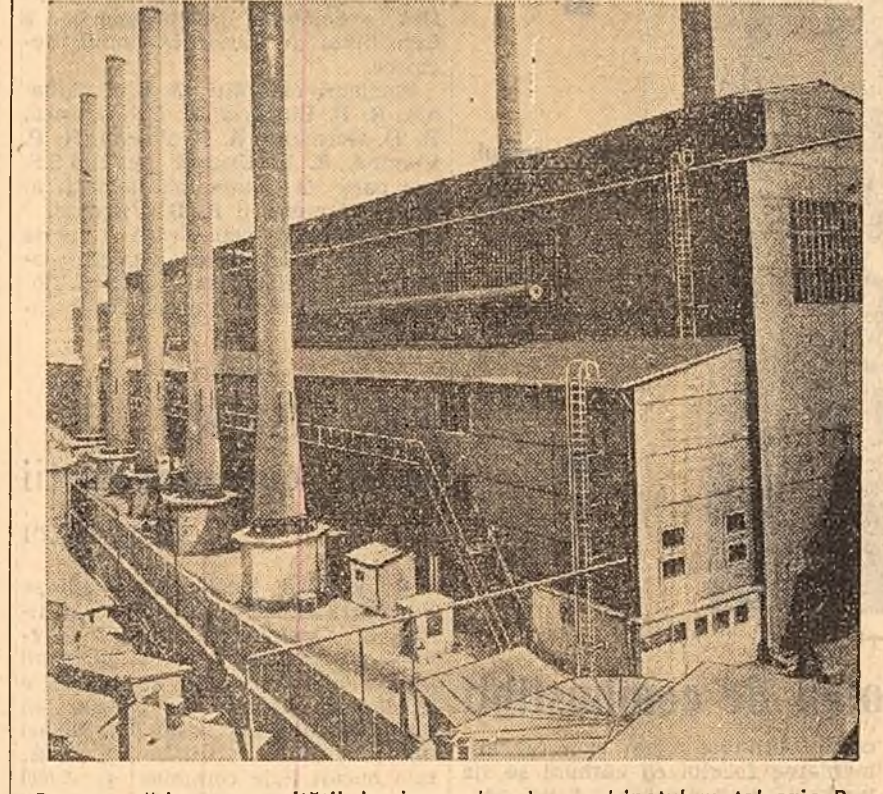
Pe mărirea capacității laminoarelor, la combinatul metalurgic Reșița s-a construit, cu ajutorul documentației tehnice sovietice, cupatoarele edinci de la laminoarele combinatului. În fotografie: Aspect exterior al cupatoarelor adinci (Foto Gh. Vințilă)
