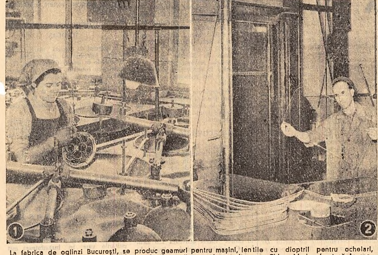
La fabrica de oglinzi București, se produc geamul pentru mașini, lentilele cu dioptrii pentru ochelari, geamul curbat pentru vitrine etc. În fotografia nr. 1 muncitorii Chisu Maria, frunțaș în realizarea de economii, lucrînd la mașina de șlefuit lentile; iar în fotografia nr. 2, muncitorii Constantin Dilimo, verificînd cum au fost șlefuite parbrizele de autocamion înainte de tratarea lor termică. (Foto R. Costin)
