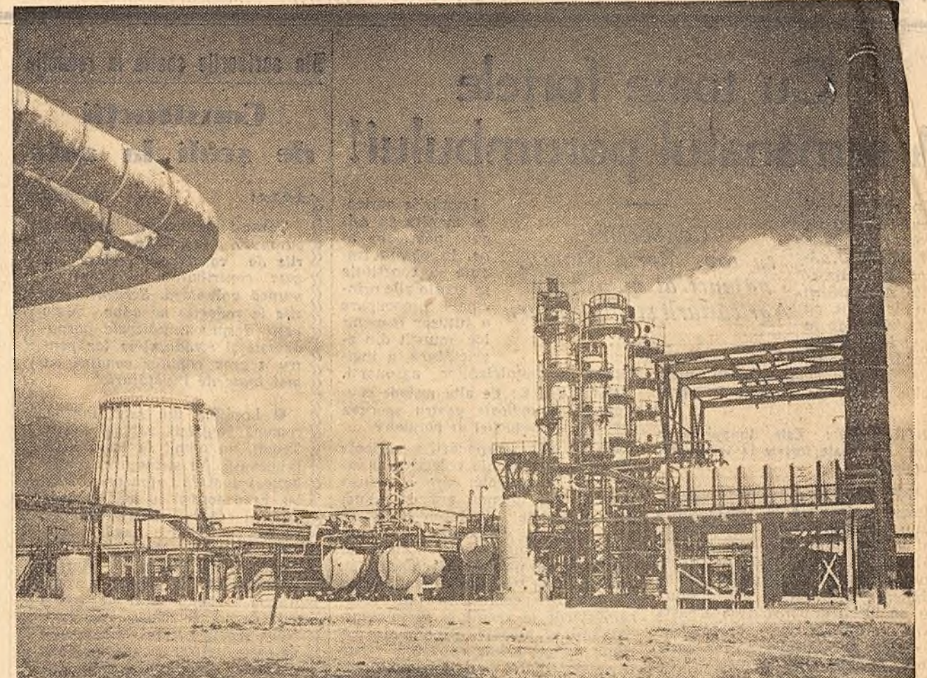
Aspect exterior al instalației D.A.V.-2 pentru obținerea de uleiuri superioare și benzină de la Blocul de ulei Teleajen. (Foto Gh. Vinții)
