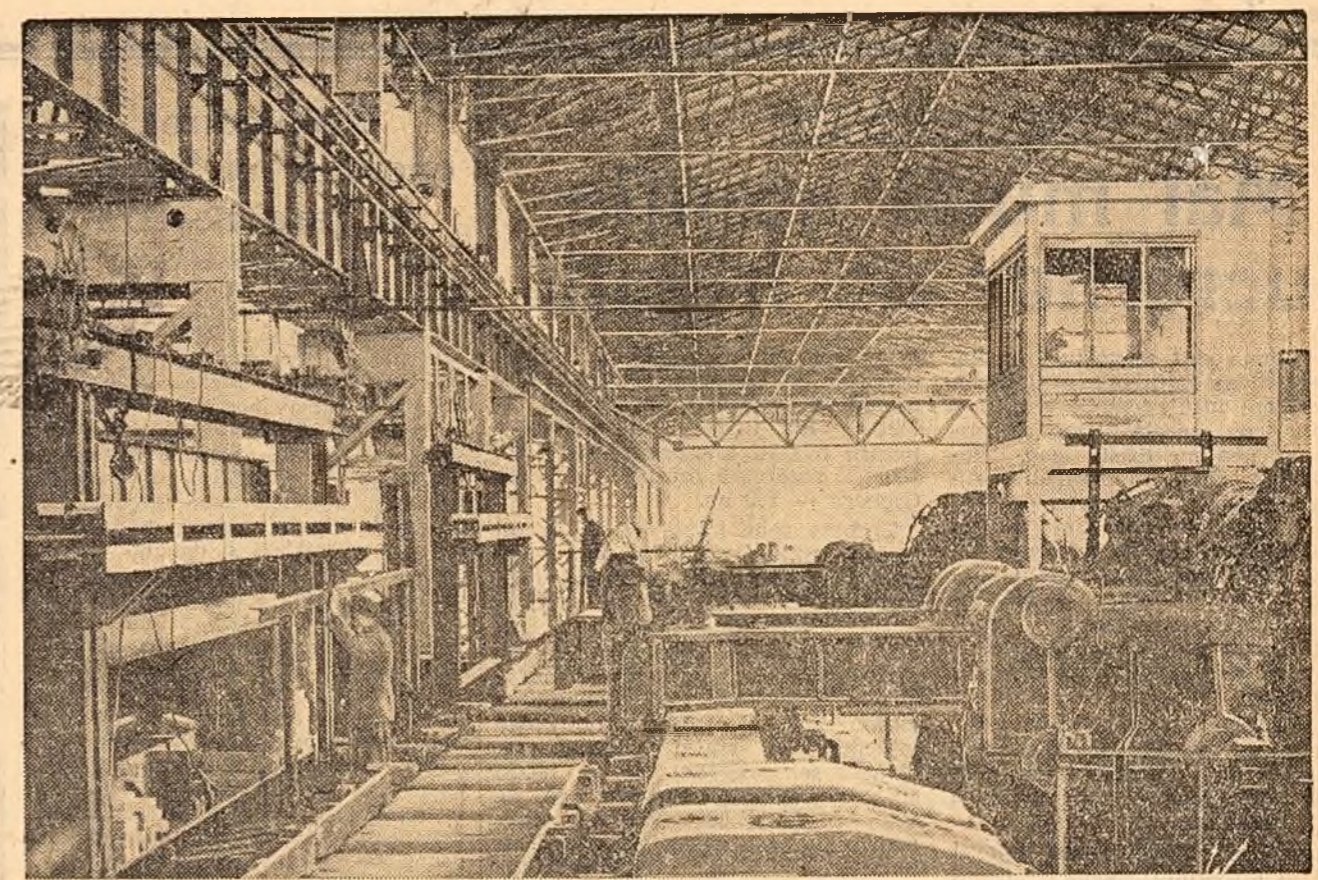
La Combinatul siderurgic Hunedoara continuă lucrările de montare a laminorului de 650 milimetri. În fotografie, cala cu role pentru alimentarea cuptoarelor. (Foto Gh. Vințilă)
