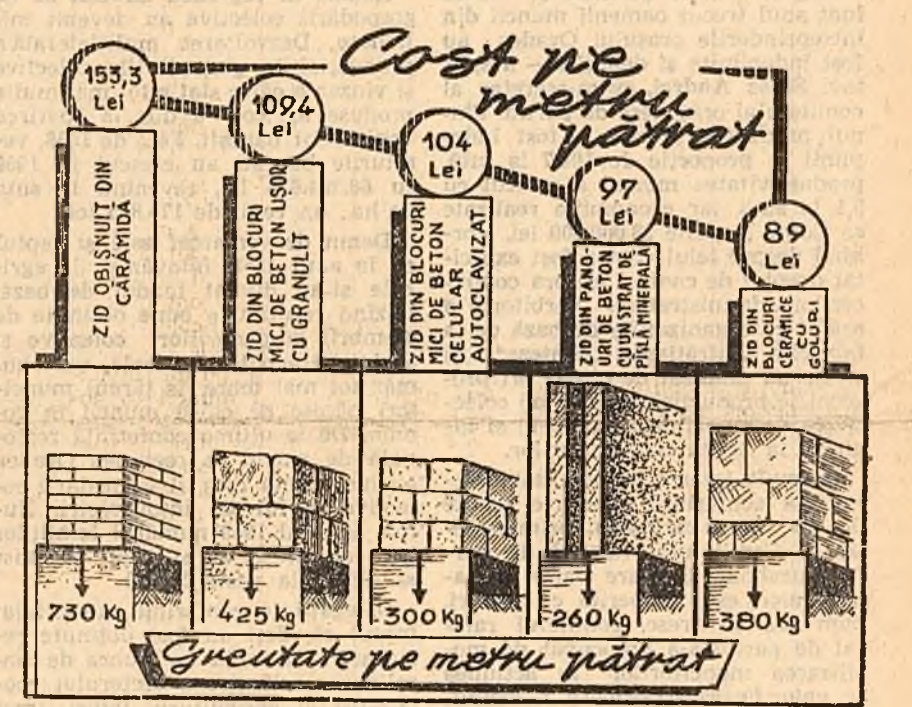
Graficul redă cîteva din avantajele mari pe care le prezintă folosirea noilor materiale de construcții față de materialele clasice — cărămida, betonul etc. — Așa cum reiese din grafic, introducerea noilor materiale de construcții asigură scăderea prețului de cost pe metru pătrat de zidărie și în plus duce la scăderea simțitoare a greutății construcției. (Citiți în pagina II-a „Cale liberă — materialelor noi de construcții”).
