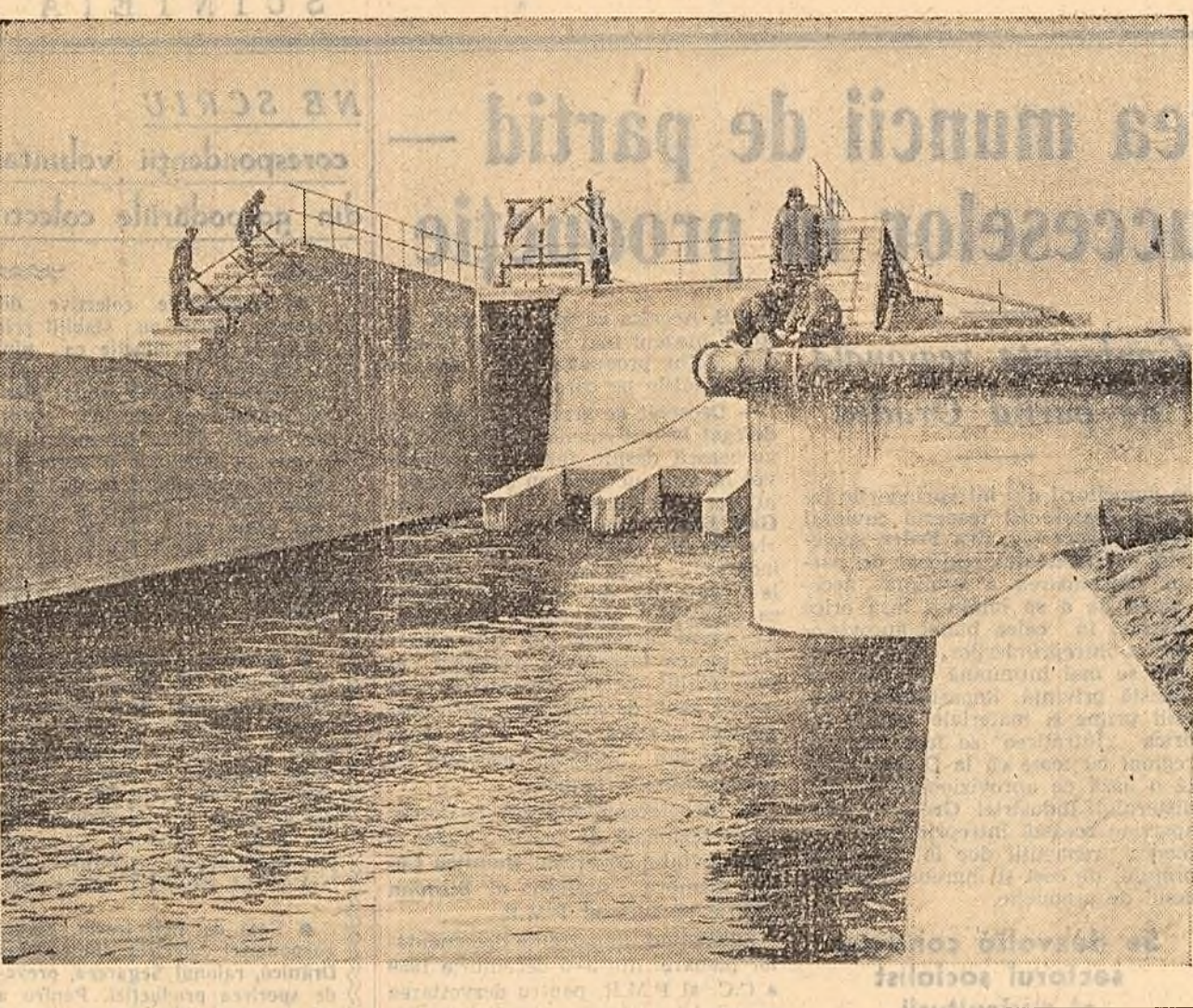
Șantierul de la Cernica. Aici s-a amenajat un lac de acumulare cu o suprafață de 360 hectare, ce va servi la irigația unei mari întinderi de teren agricol. În fotografie: Stăvilarul din mijlocul gîntului.
