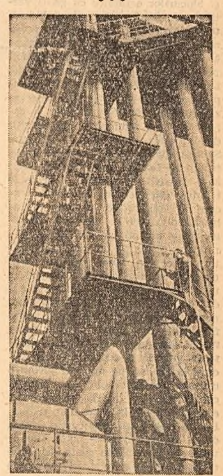
Uzinele „21 Decembrie” din Copșa Mică. Răcitorul tubular de gaze. Instalația valorifică zincul din zgură.
