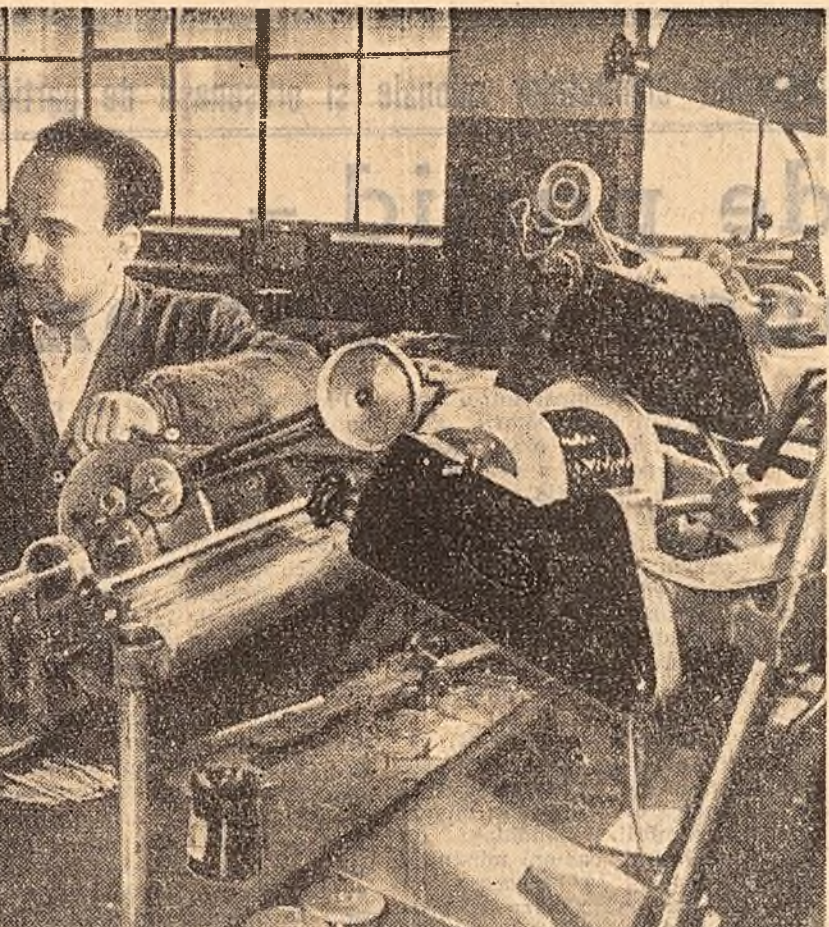
Pe șantierul de la Roznov: Fabrica de azotă de amoniu. (Foto: R. Costin)
