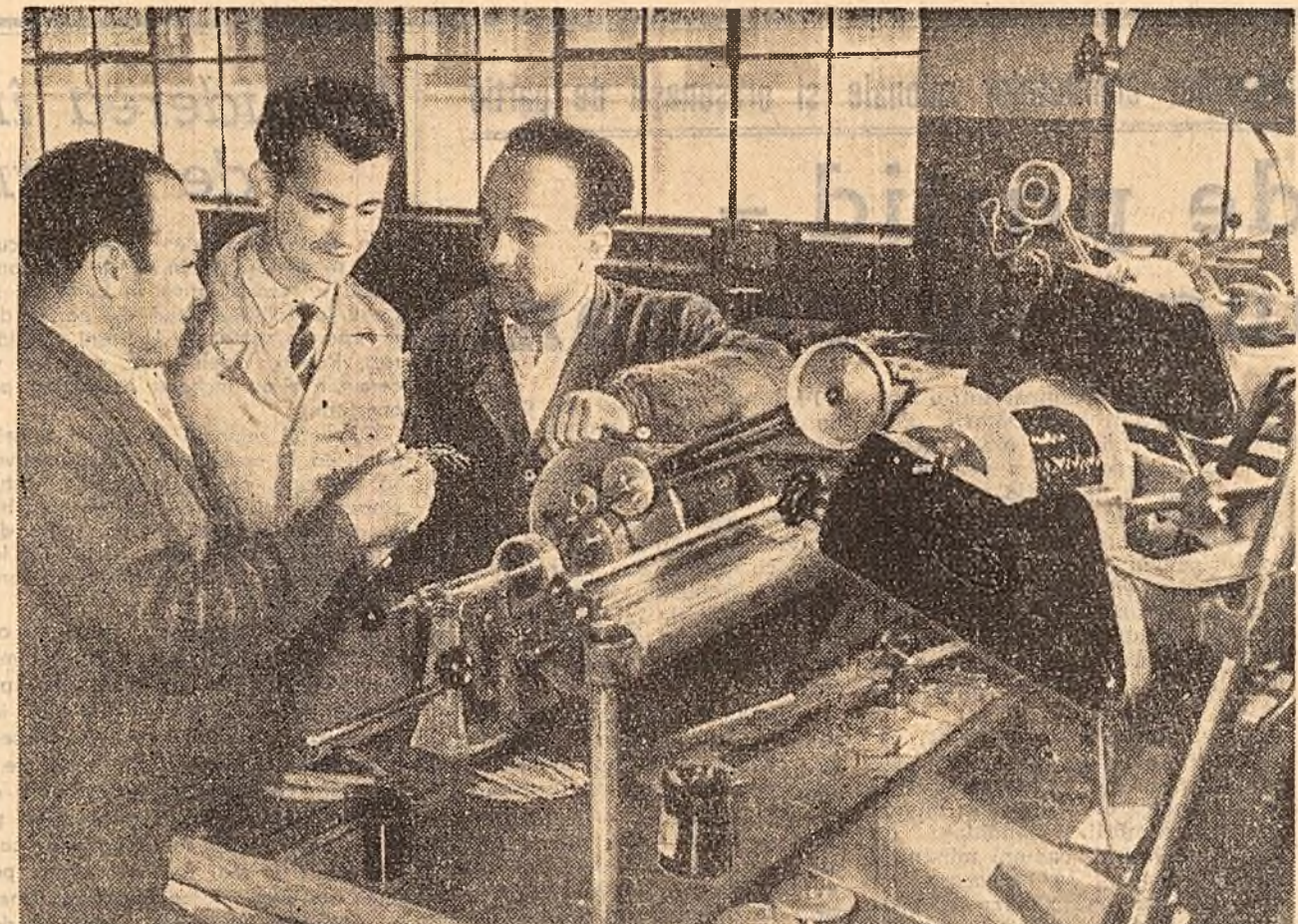
La uzinele „Grigore Preoteasa”. Șeful de echipă Mircea Coman discutînd cu montorul Axenia Anghel și maestrul Dumitru Nicolae din cadrul atelierului de bobinaj despre calitatea unei bobine de transformator de la o stație de 150 vați. Această echipă s-a angajat să depășească zilnic planul de producție și să realizeze numai produse de bună calitate. (Foto Agerpres)
