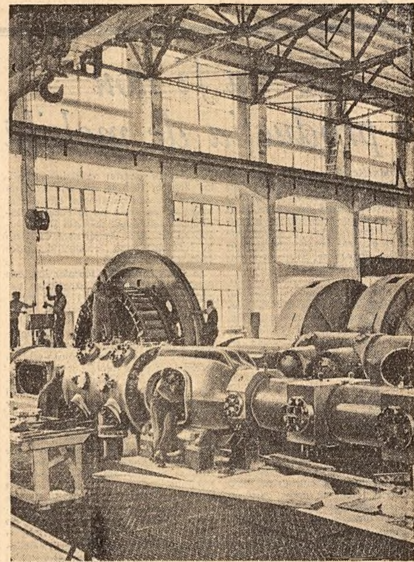
Combinatul de îngreșăminte azotoase Roznov. În secția de amoniac se montează compresoarele pentru gaz convertit, fiecare cu o capacitate de 16.500 m.c. pe oră. În fotografie: Echipa condusă de Eugen Birsan, lucrînd la montarea acestor compresoare.
