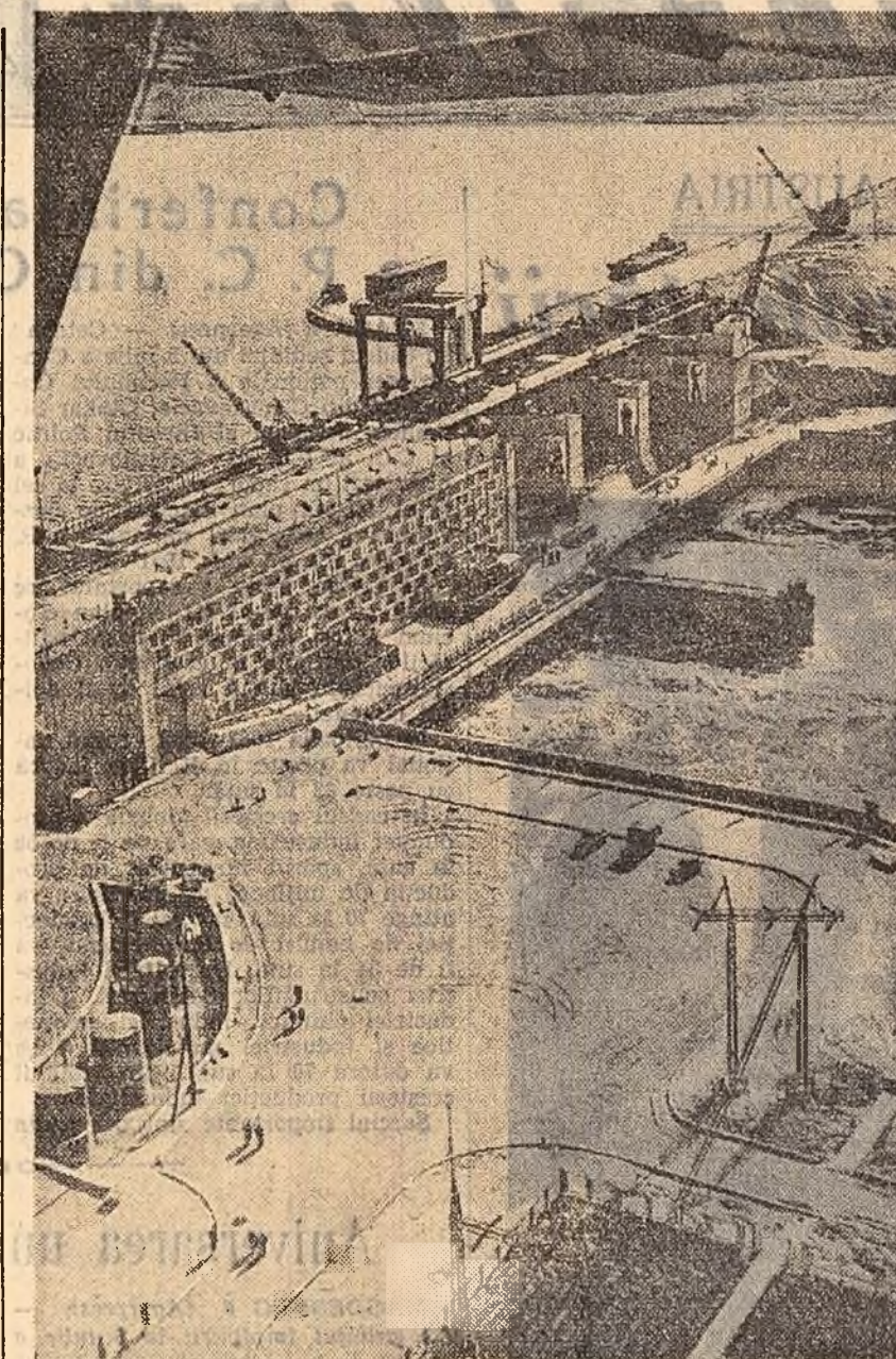
Aspect de pe șantierul hidrocentralei de la Kaunas (R.S.S. Lituaniană), pe râul Nemun
