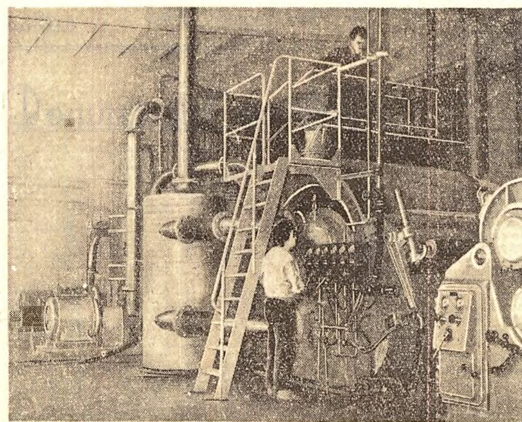
Dacă în fotografie se văd numai doi oameni, aceasta se datorește și faptului că procesul de producție este în cea mai mare parte automatizat. În fotografie: Mașina „Presbat” unde se trag iolile de celuloză albită.
