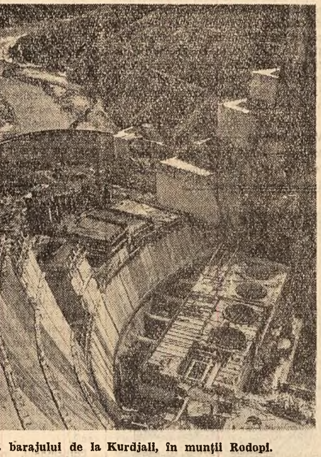
Construcția barajului de la Kurdjall, în munții Rodopi.
