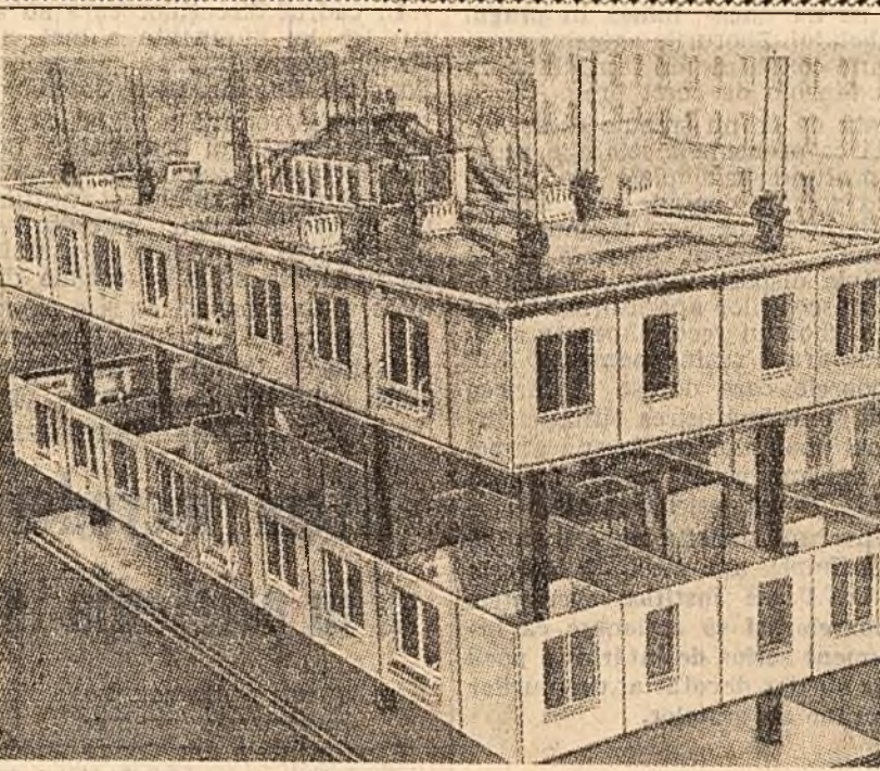
Casa „crește”... de sus în jos. După ce a fost montat etajul IV, a început ridicarea etajului III.
