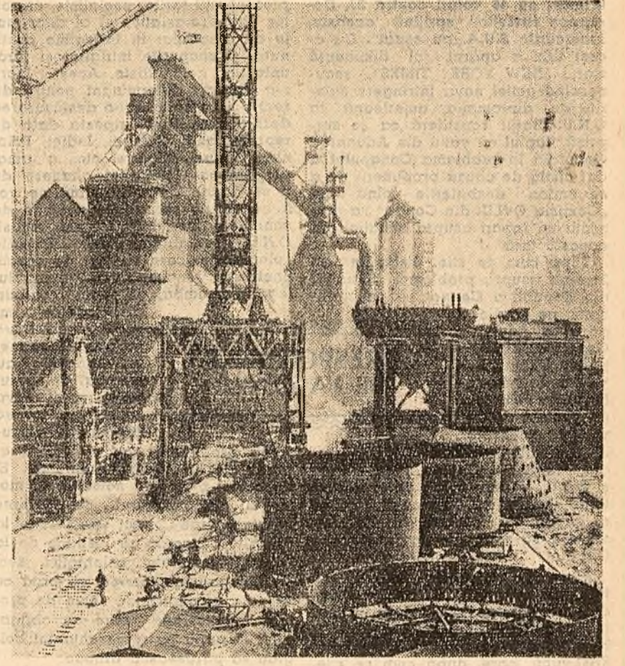
Furnal în construcție la uzina siderurgică „V. I. Lenin” din Kriivoi-Rog (U.R.S.S.)
