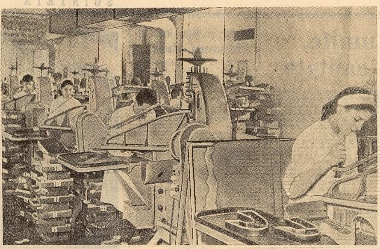
La întreprinderea „Kirov” din Capitală, a intrat în funcțiune recent o nouă secție de croit fețe mecanic prin ștanțare. Prin intrarea în producție a acestei noi secții, productivitatea muncii crește simțitor. În fotografie: noua secție. (Foto M. Cioe)
