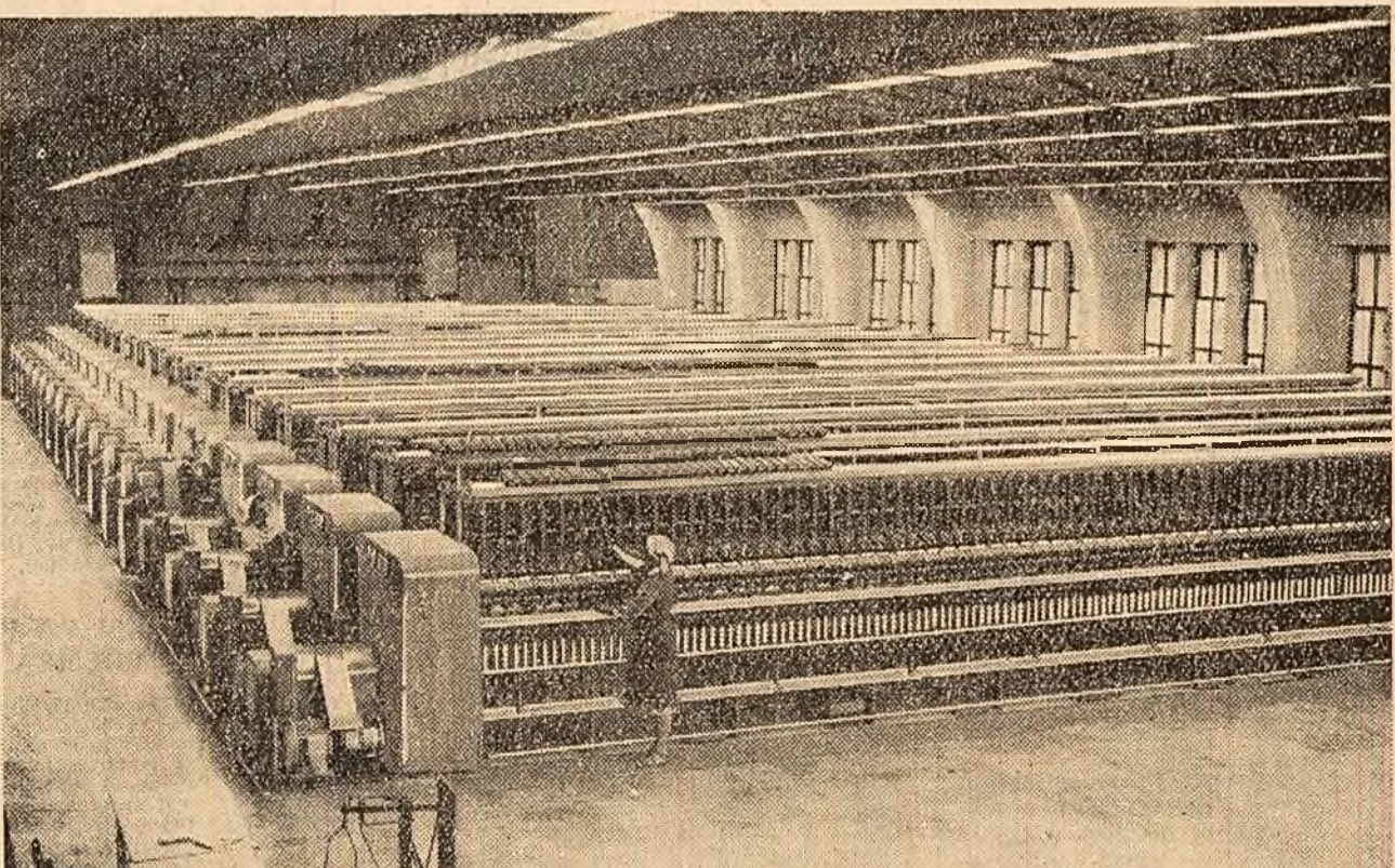
Noua filatură din cadrul fabricii de postav Buhuși este înzestrată cu utilaj modern de înaltă productivitate. În fotografie: Vedere interioară a secției de ringuri din noua filatură. (Foto Agerpres)
