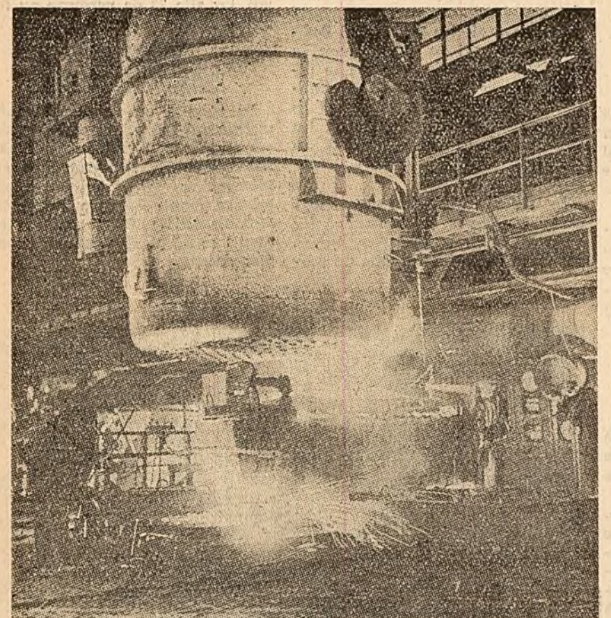
La sfîrșitul septenaliului, producția uzinel siderurgice din Novo-Lipețk (U.R.S.S.), calculată pe cap de muncitor, va fi aproape dublă față de cea obținută în cele mai bune zile din S.U.A. În cișeu: o instalație de turnare continuă a oțelului — una din cele mai mari din lume.
