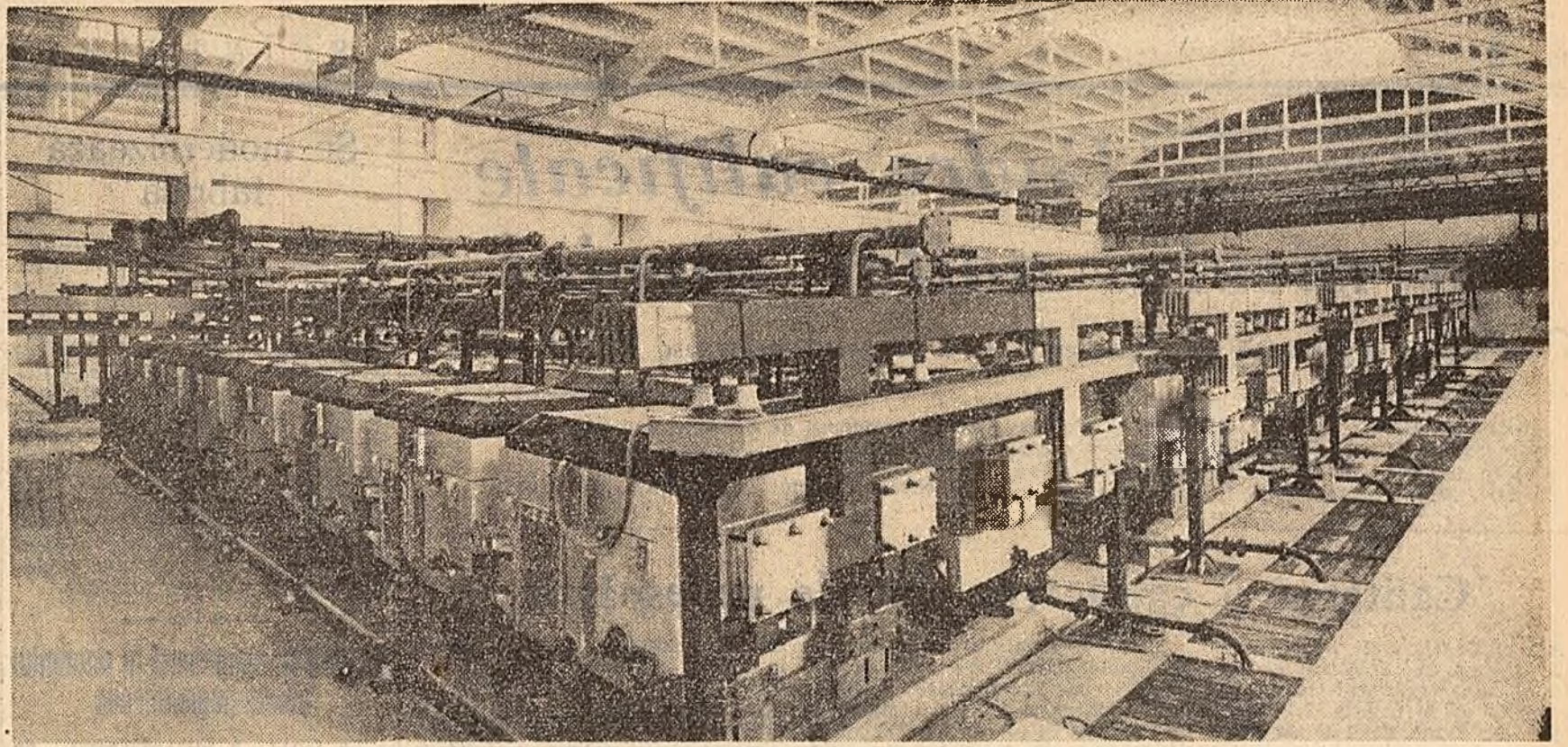
Aspect interior al secției de electroliză de la noul Combinat chimic din Borzsei.
