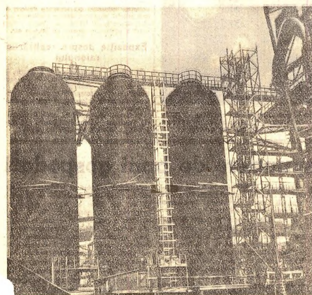
REȘIȚA: Cauperele unuia din furnalele aflate în reconstrucție.
