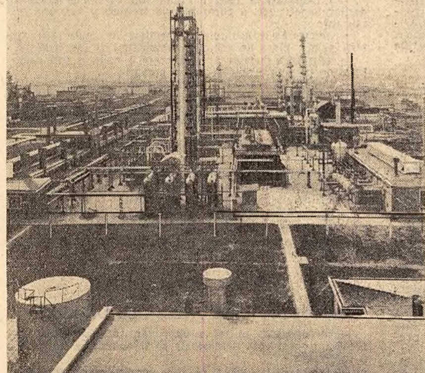
Rafinăria nr. 10—Onești, construită în anii puterii populare, se numără printre marile obiective ale industriei petroliere din țara noastră. În fotografia de față: Aspect al instalației de fracționare a gazelor de la rafinăria din Onești.
