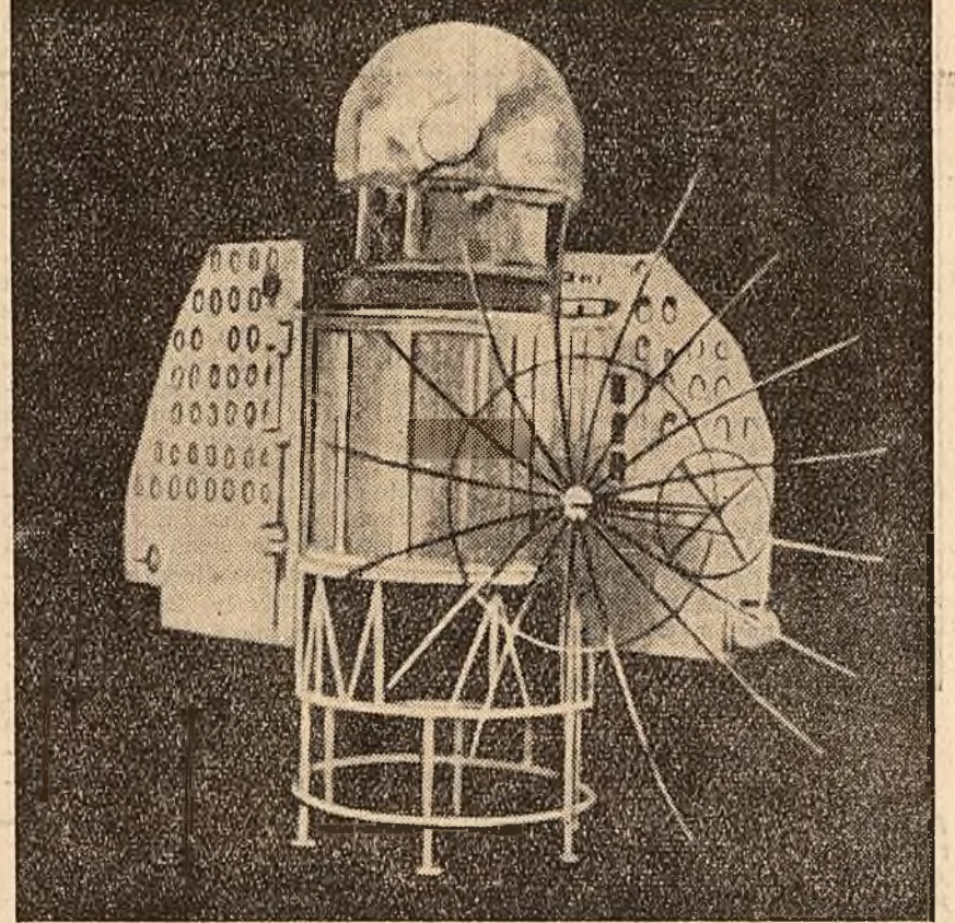
Stațiunea interplanetară automată pe suportul de montaj. Privire din spate
